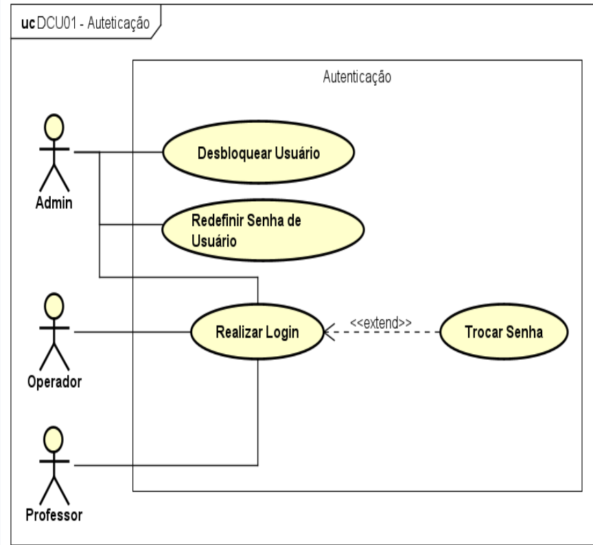
DCU01 – Autenticação
