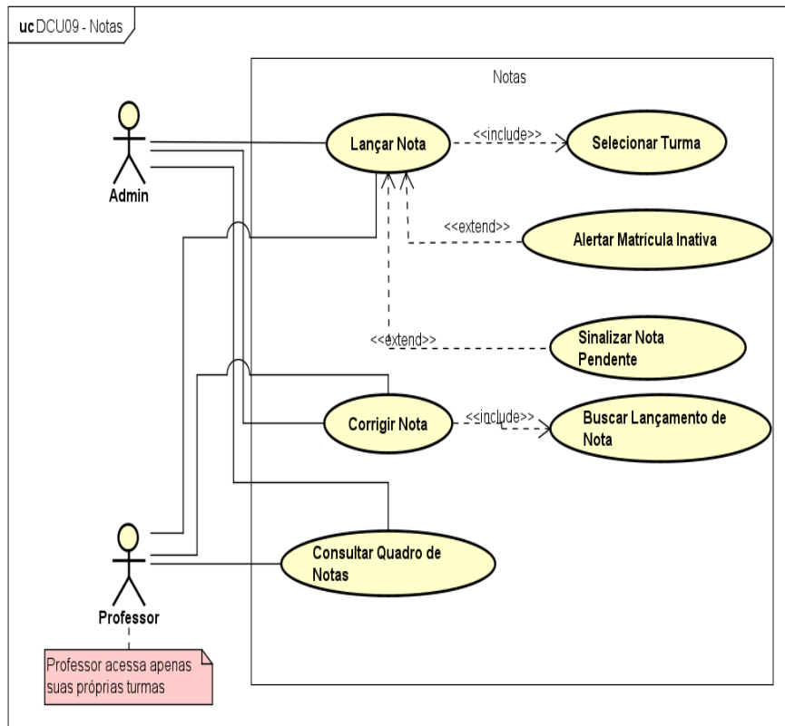
DCU09 – Notas
