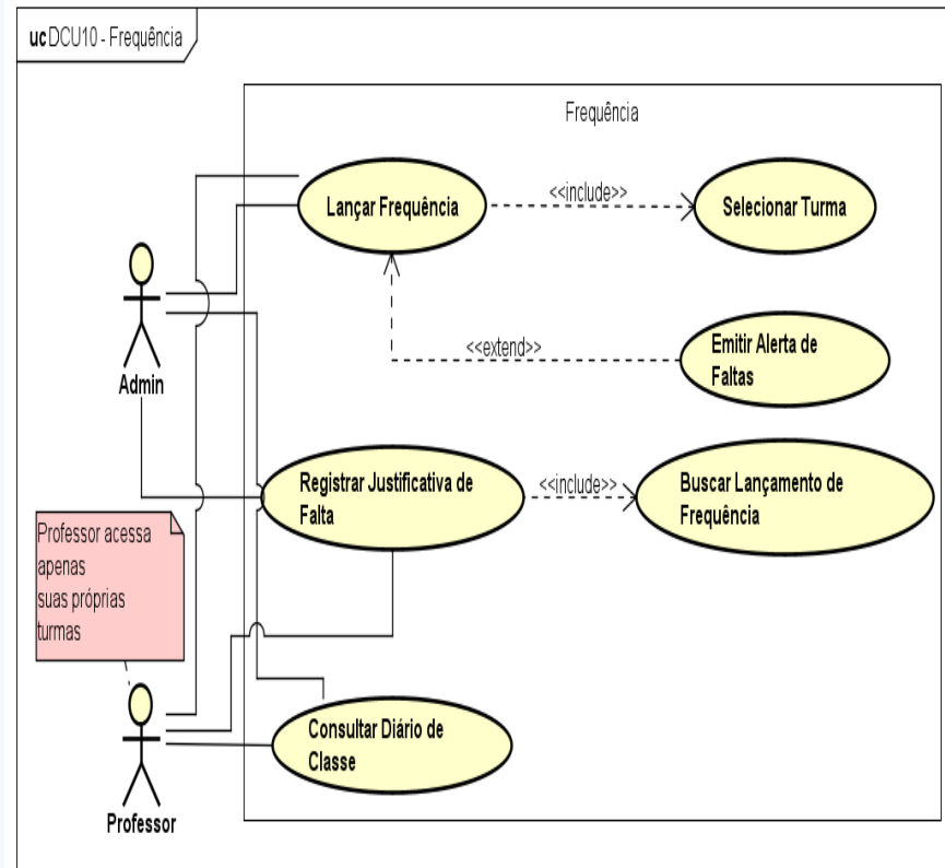
DCU10 – Frequência
