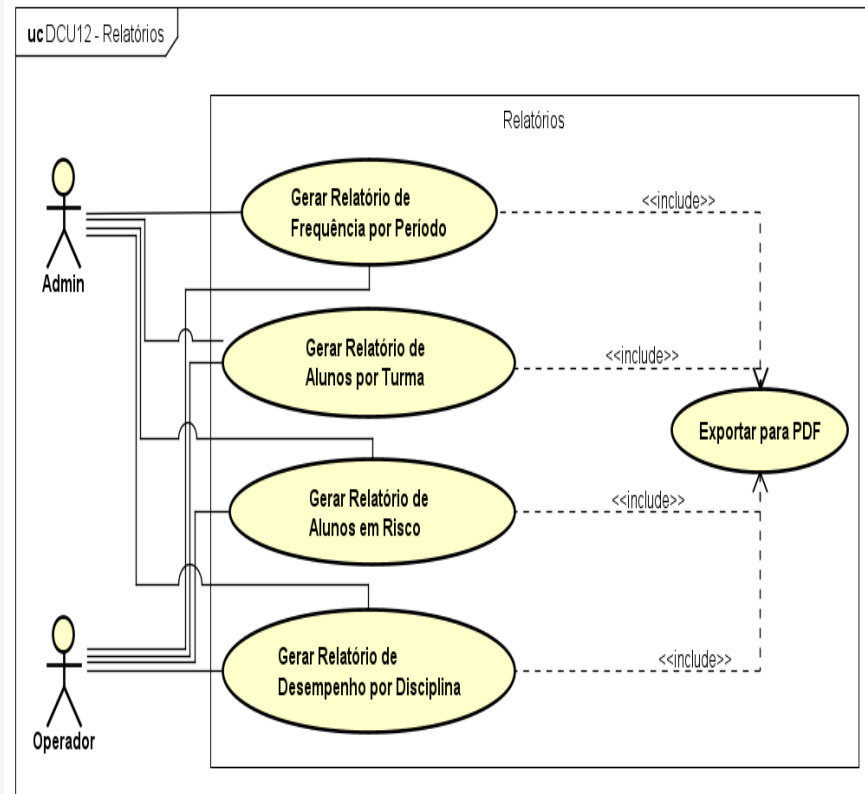
DCU12 – Relatórios
